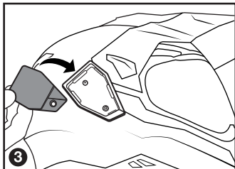
放置运动相机支架
