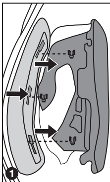
取下面颊垫
